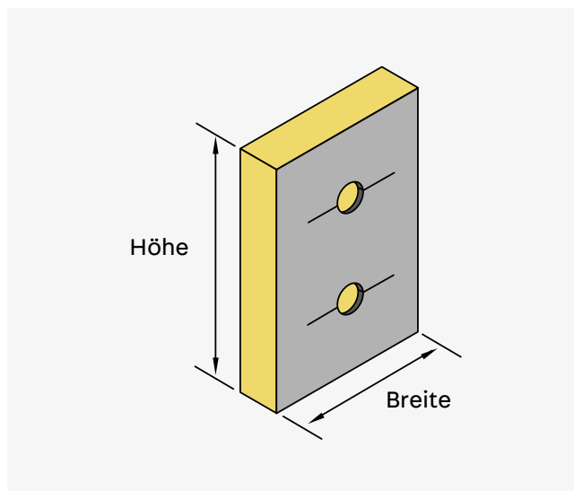
JORDAHL® Brandschutzmanschette für JDSDQ
